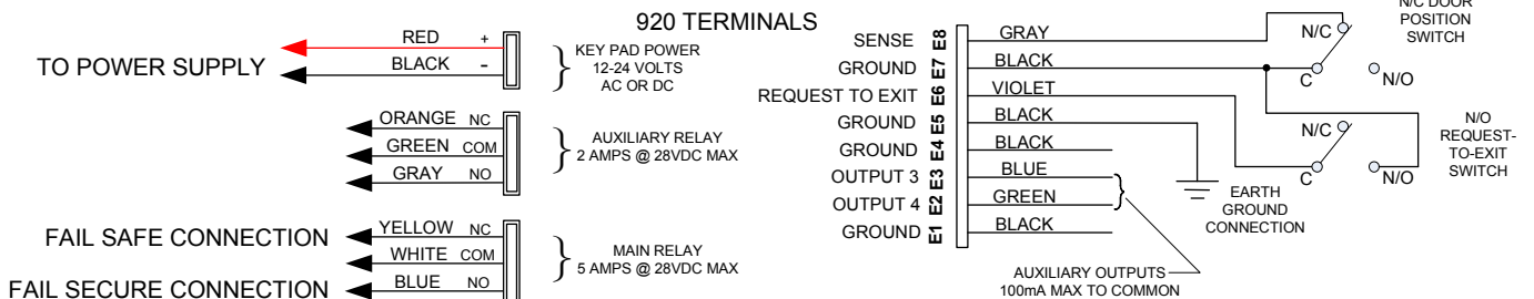
Fig. 2 Wiring Pigtail Color Code
